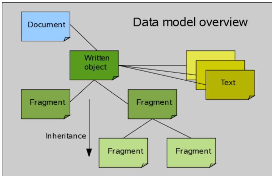
Abbildung 2: Datenmodellschema
